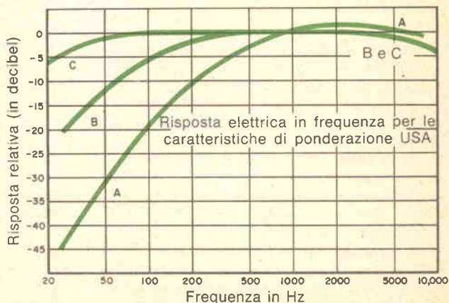
Fig. 2 - Le curve indicano le caratteristiche di risposta ponderata specificate dall'American Standard Institute.
