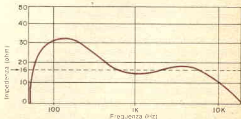
Fig. 2 - Tipica curva di impedenza per un altoparlante di tipo a larga banda; l'impedenza nominale è di 16 \Omega .
