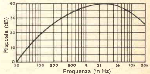
Fig. 2 - La risposta del filtro segue la curva di ponderazione A della ASA ed è prolungata alle alte frequenze secondo le curve di Fletcher-Munson.
